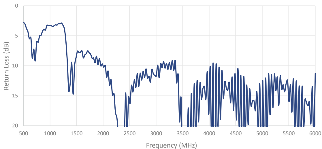
Cable 4: 5GNR
