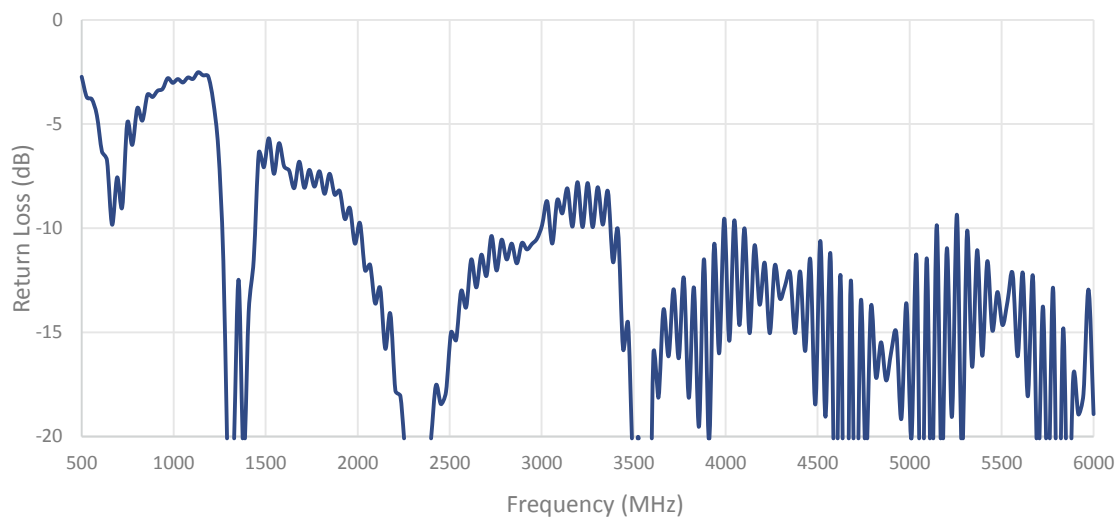
Cable 2: 5GNR
