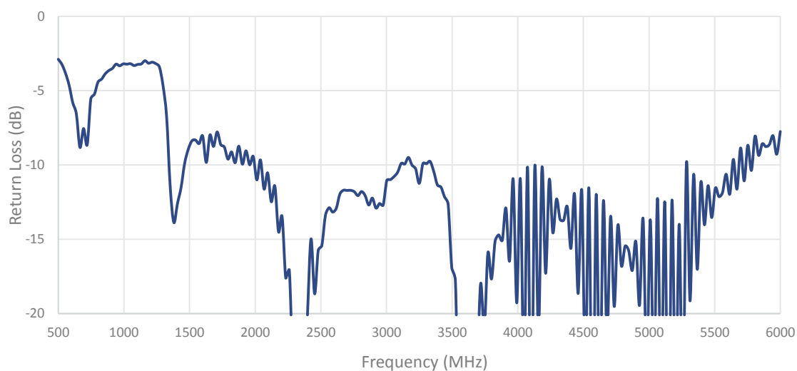
Cable 3: 5GNR
